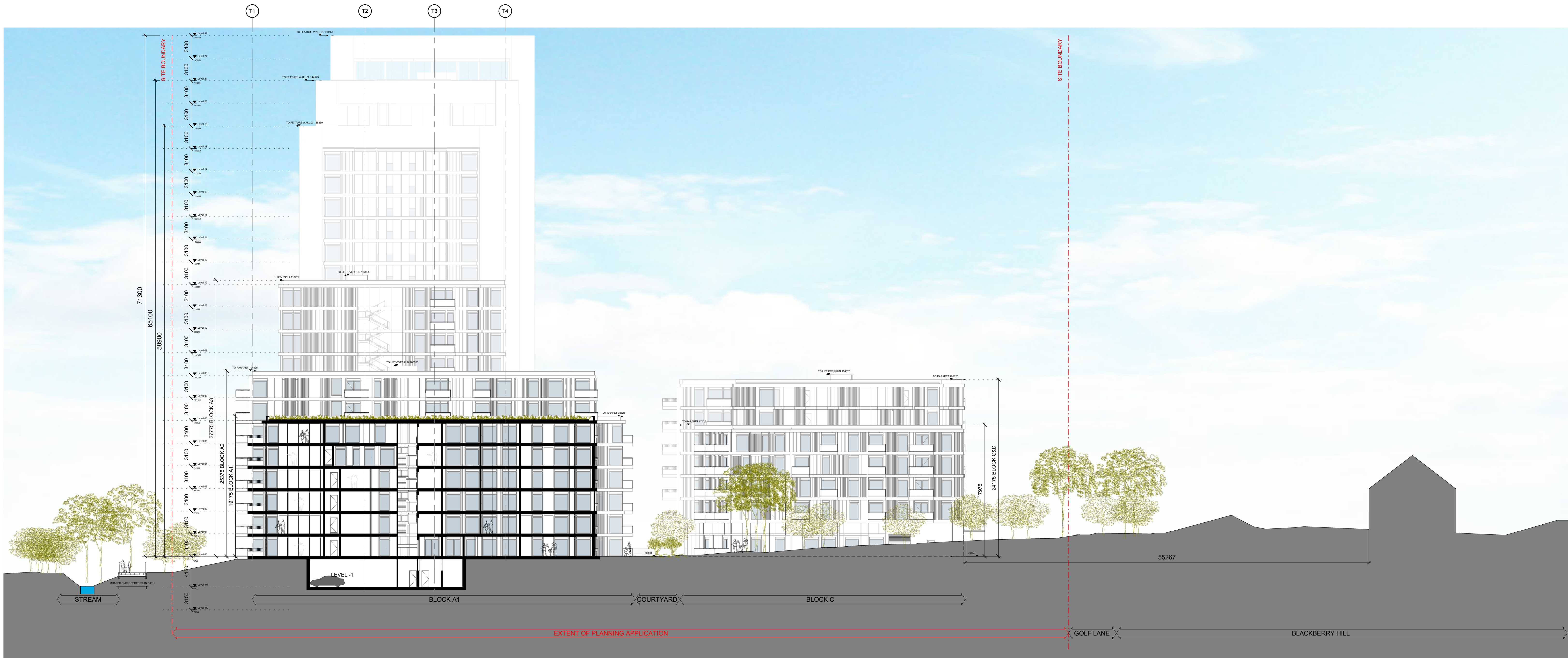
2 Site Section 04 1 : 250
